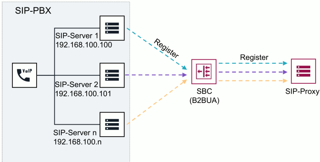
Abbildung 2: Redundanz im Registrierungsmodus
