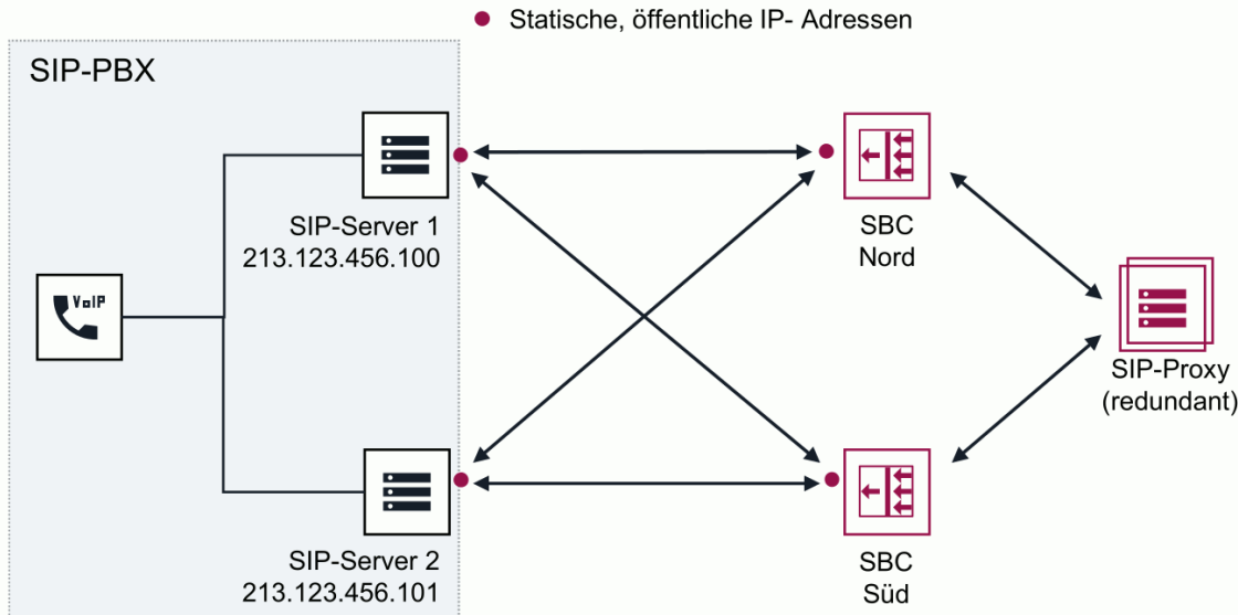
Abbildung 3: Statische SIP Trunk Kopplung (Darstellung des redundanten Szenarios)
