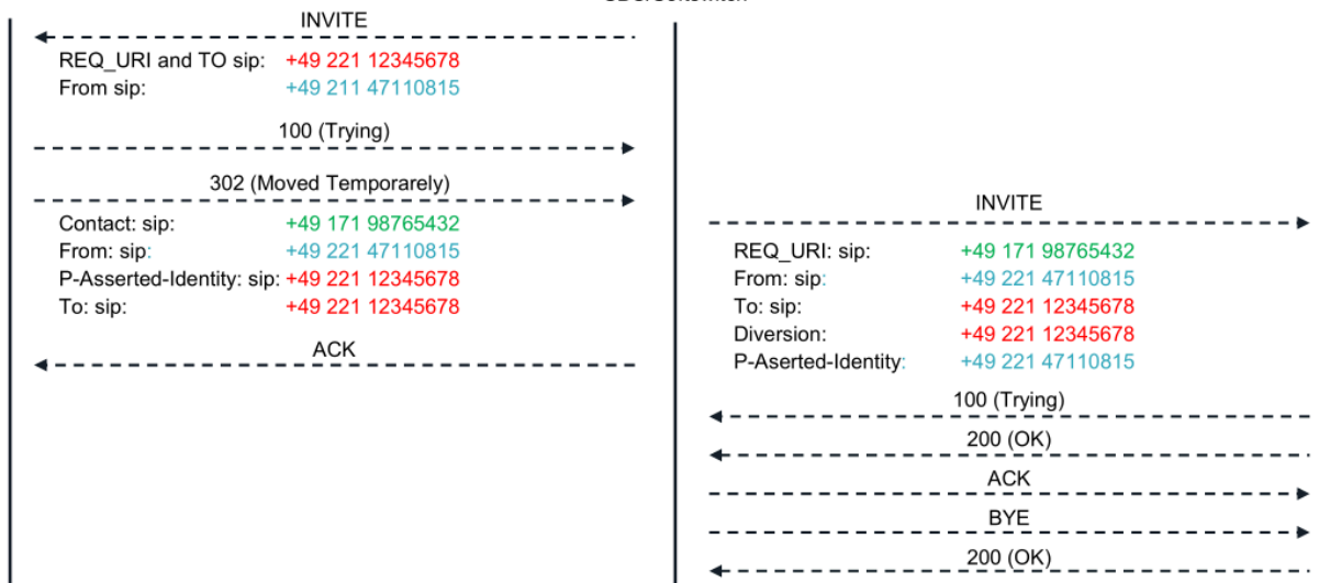
Abbildung 6: Rufumleitung mit 302 Moved Temporarily
