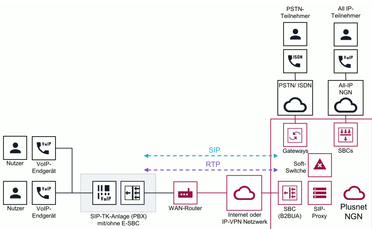
Abbildung 1: Vereinfachtes Netzdiagramm
