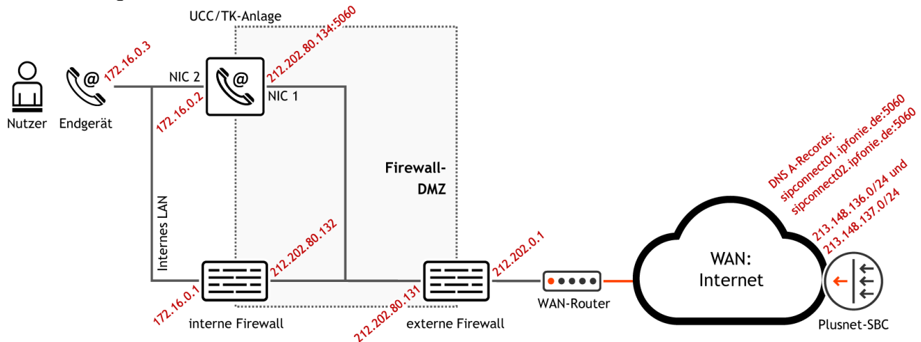
Abbildung 8: Erste sinnvolle IP-Topologie an einem Internet-Uplink im fix-IP-Modus
