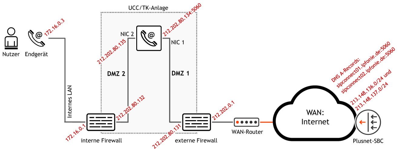
Abbildung 9: Zweite sinnvolle IP-Topologie an einem Internet-Uplink im fix-IP-Modus
