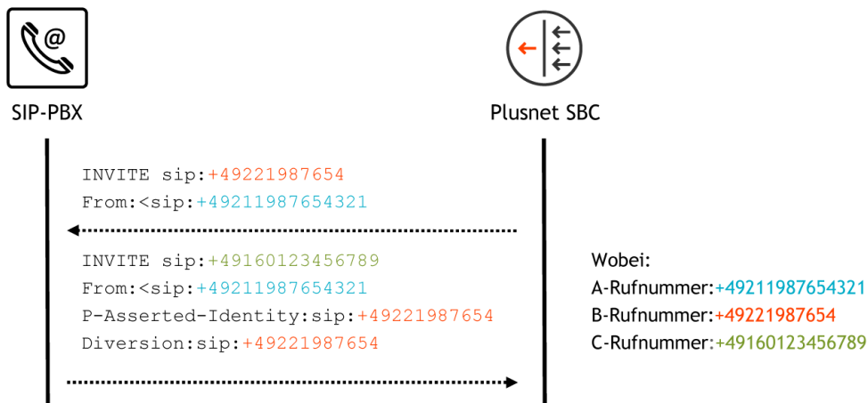
Abbildung 5: Call Forward
