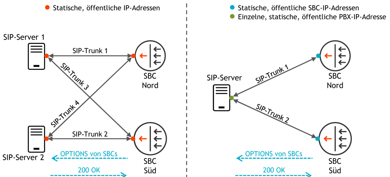
Abbildung 4: Redundanz im Peering Modus
