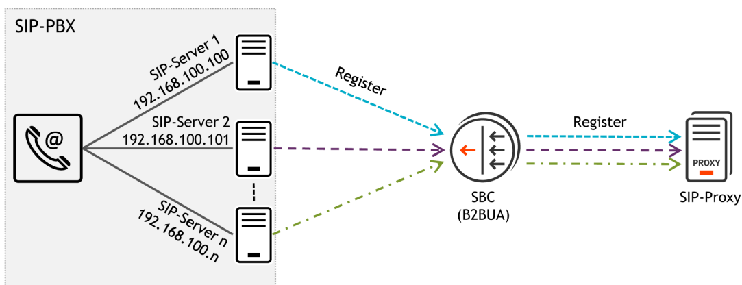
Abbildung 2: Redundanz im Registrierungsmodus
