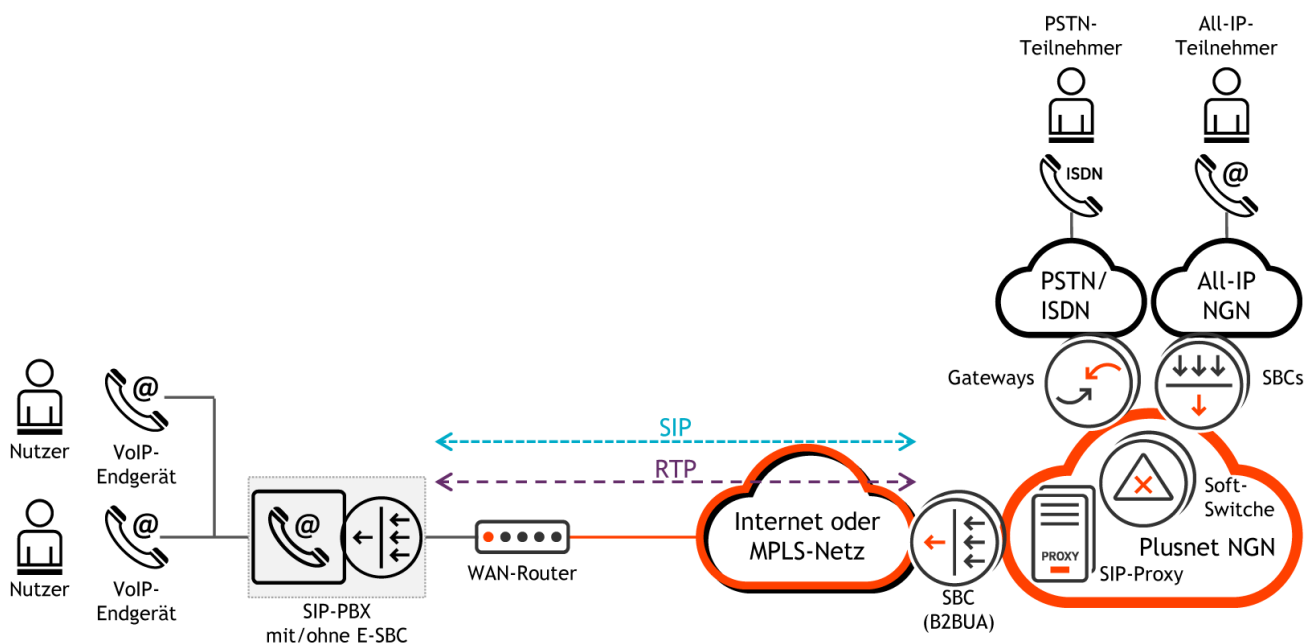
Abbildung 1: Vereinfachtes Netzwerkdiagramm
